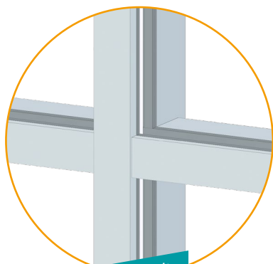
中梃连接
