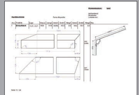
Nářez pro oplechování
