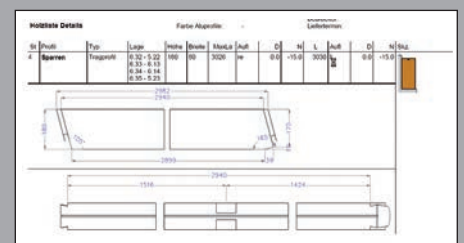
Dřevěný profil s rybinovým spojem
