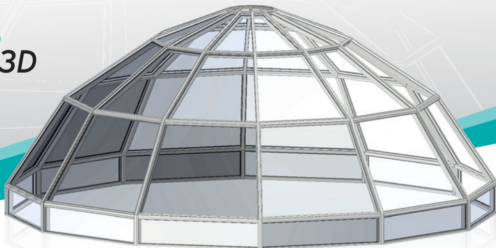
3D prikaz konstruisanja kupole
